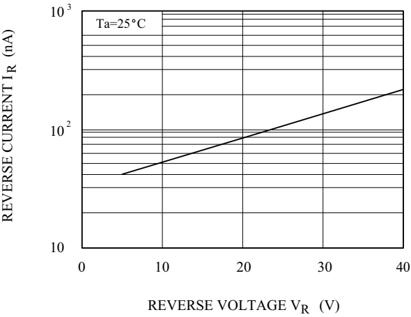
I_R - V_R
