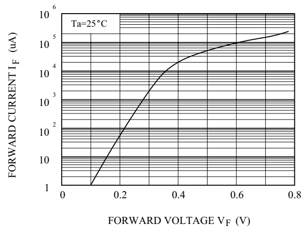
I_F - V_F
