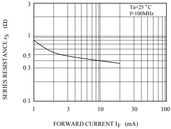
r_S - I_F
