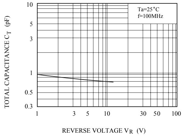
C_T - V_R
