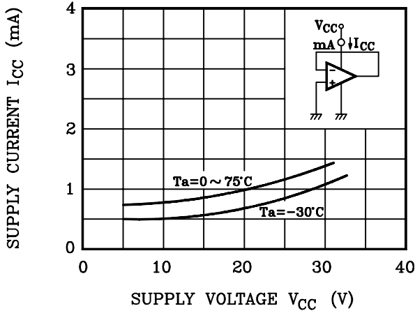
V_{CC} - I_{CC}
