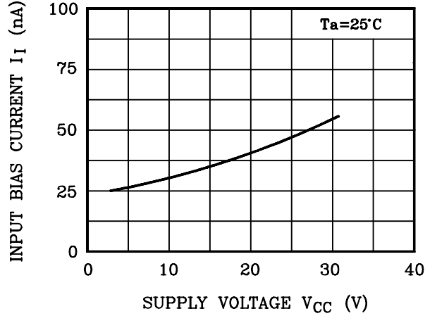
V_{CC} - I_I
