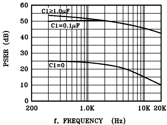
FIGURE4-C2=10 \mu F
