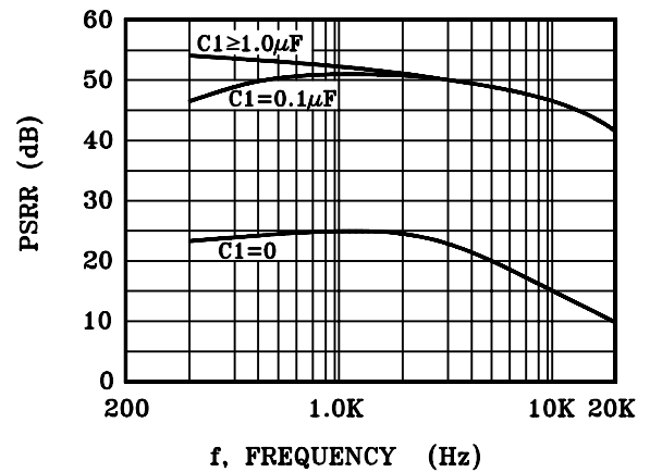
FIGURE5-C2=5.0 \mu F
