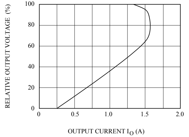
Fig.4 I_O - V_O
