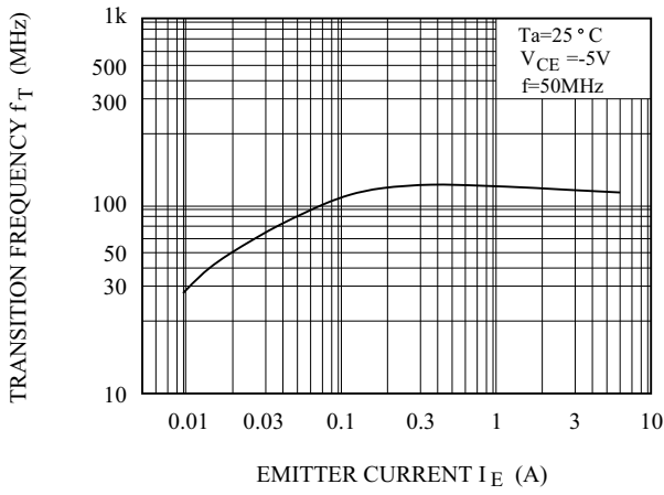
f_T - I_E
