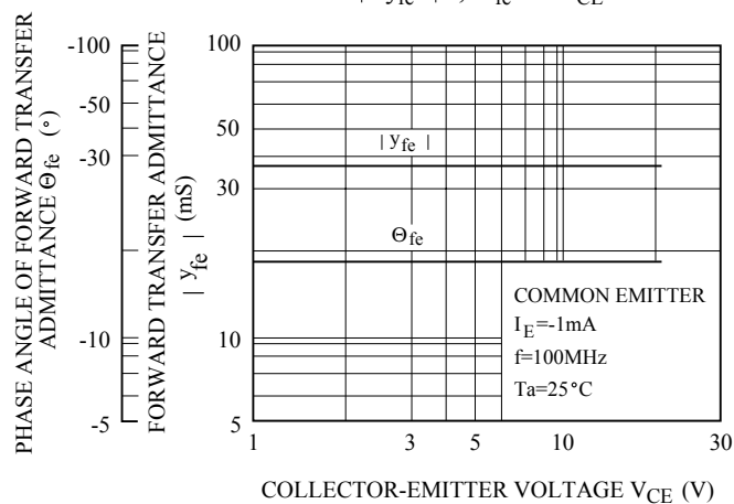
|y_{fe}|, \theta_{fe} - V_{CE}
