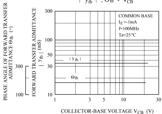
|y_{fb}|, \theta_{fb} - V_{CB}
