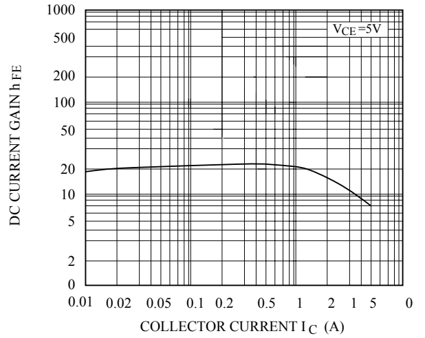
h_{FE} - I_C
