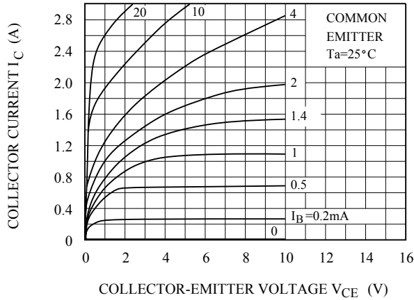
I_C - V_{CE}
