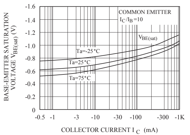
V_{BE(sat)} - I_C
