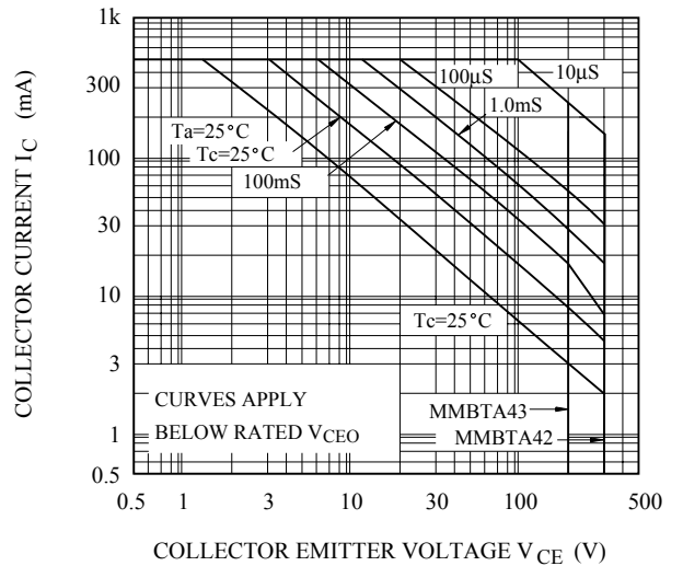
I_C - V_{CE}
