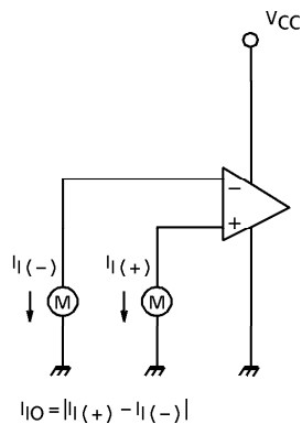
(2) I_I, I_{IO}
