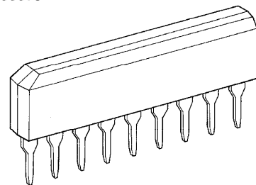
SIP9-P-2.54A
