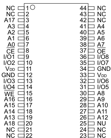
(TC55V8512FTI)
