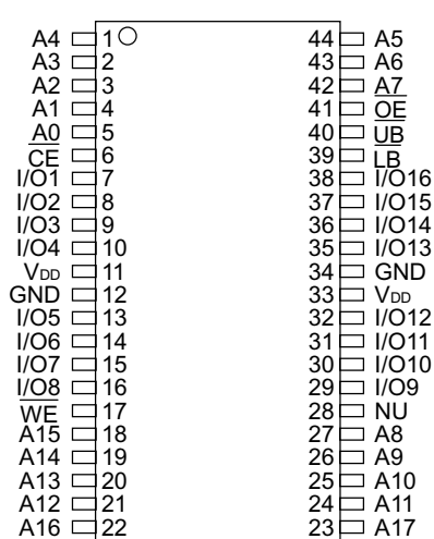
(TC55VZM216AFTI)
