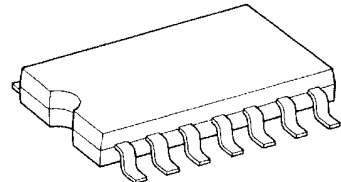
SOP14-P-300-1.27
