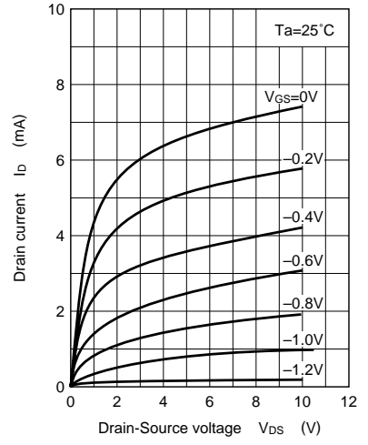
I_D - V_{DS}
