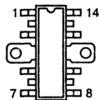
PDIP-14-1
