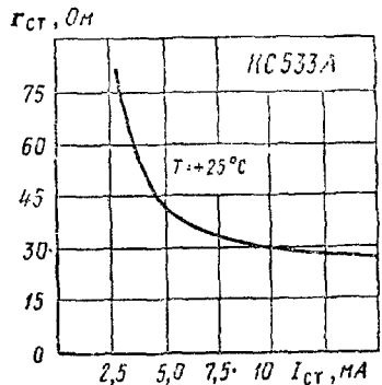
Зависимость дифференциального сопротивления от тока
