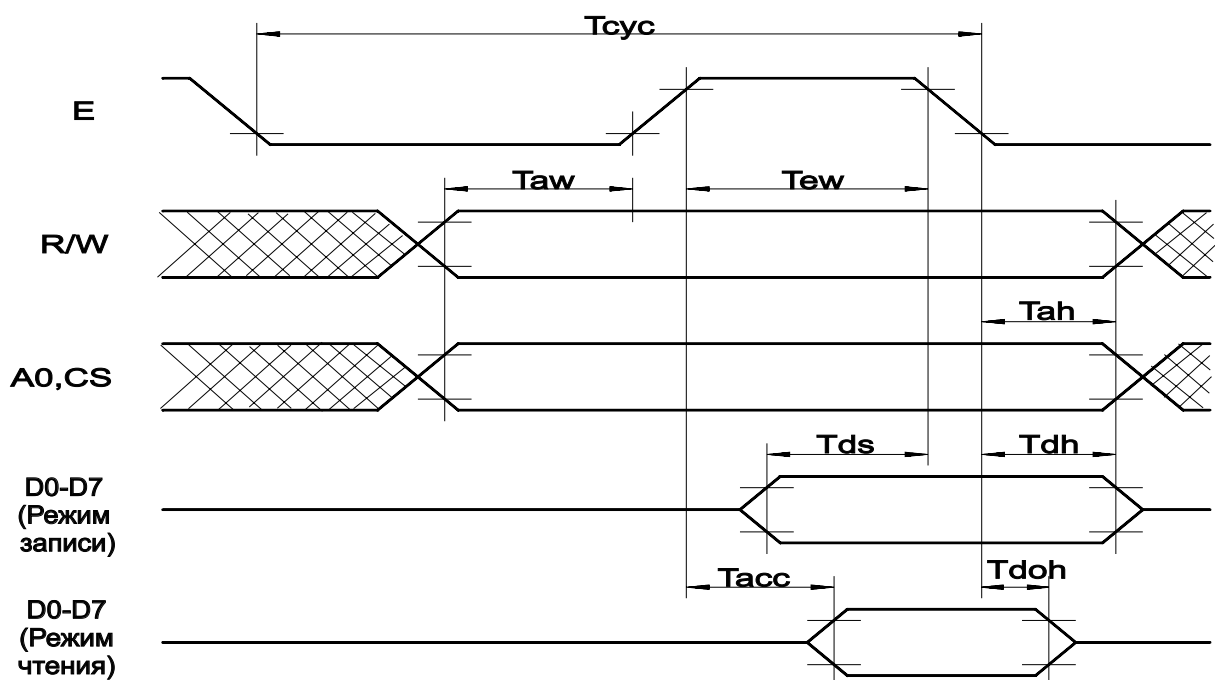
Рис. 3. Временные диаграммы протокола обмена.
