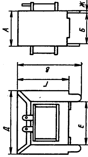
Рис. 1.2. Габаритный чертеж дросселей фильтров выпрямителей с броневым магнитопроводом
