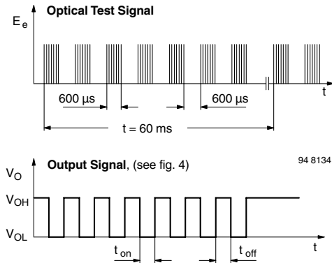
Fig. 3 - Output Function
