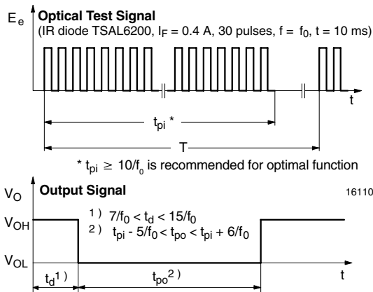
Fig. 1 - Output Function
