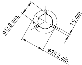
Reel hub 2:1
