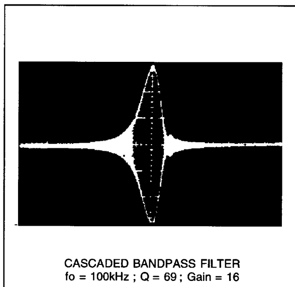
OUTPUT B
