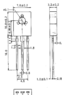
図1 JEDEC: TO-18M
