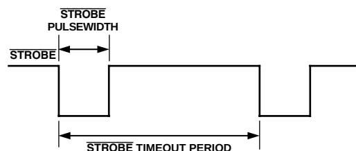
Figure 4. STROBE Parameters
