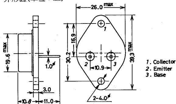
外形図(単位: mm)
