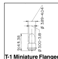
T-1 Miniature Flanged
