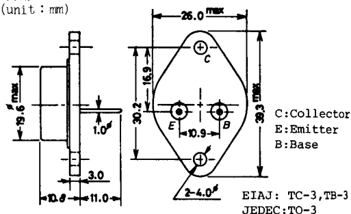
外形図 2017 (unit: mm)
