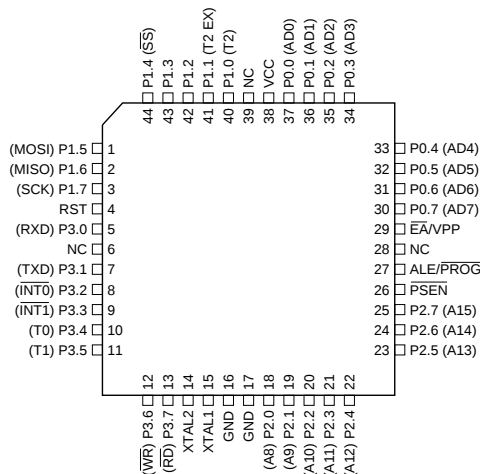
PQFP/TQFP
