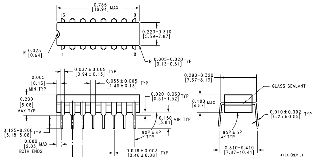
16 Lead Ceramic Dual-In-Line Package (D) NS Package Number J16A
