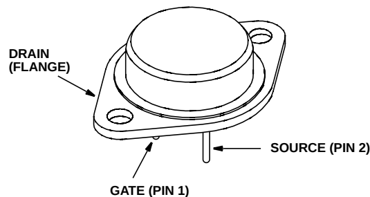
JEDEC TO-204AA
