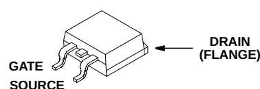
JEDEC TO-263A
