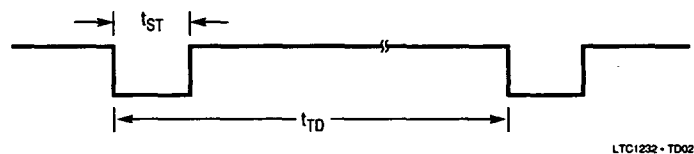
Strobe Input
