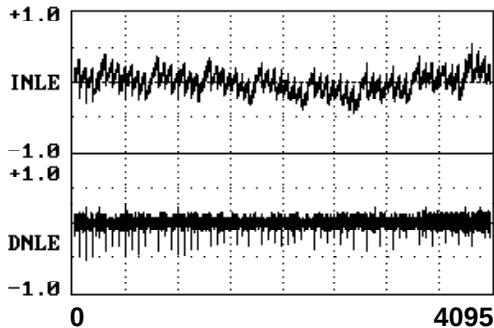
Vcc = 3.30V
