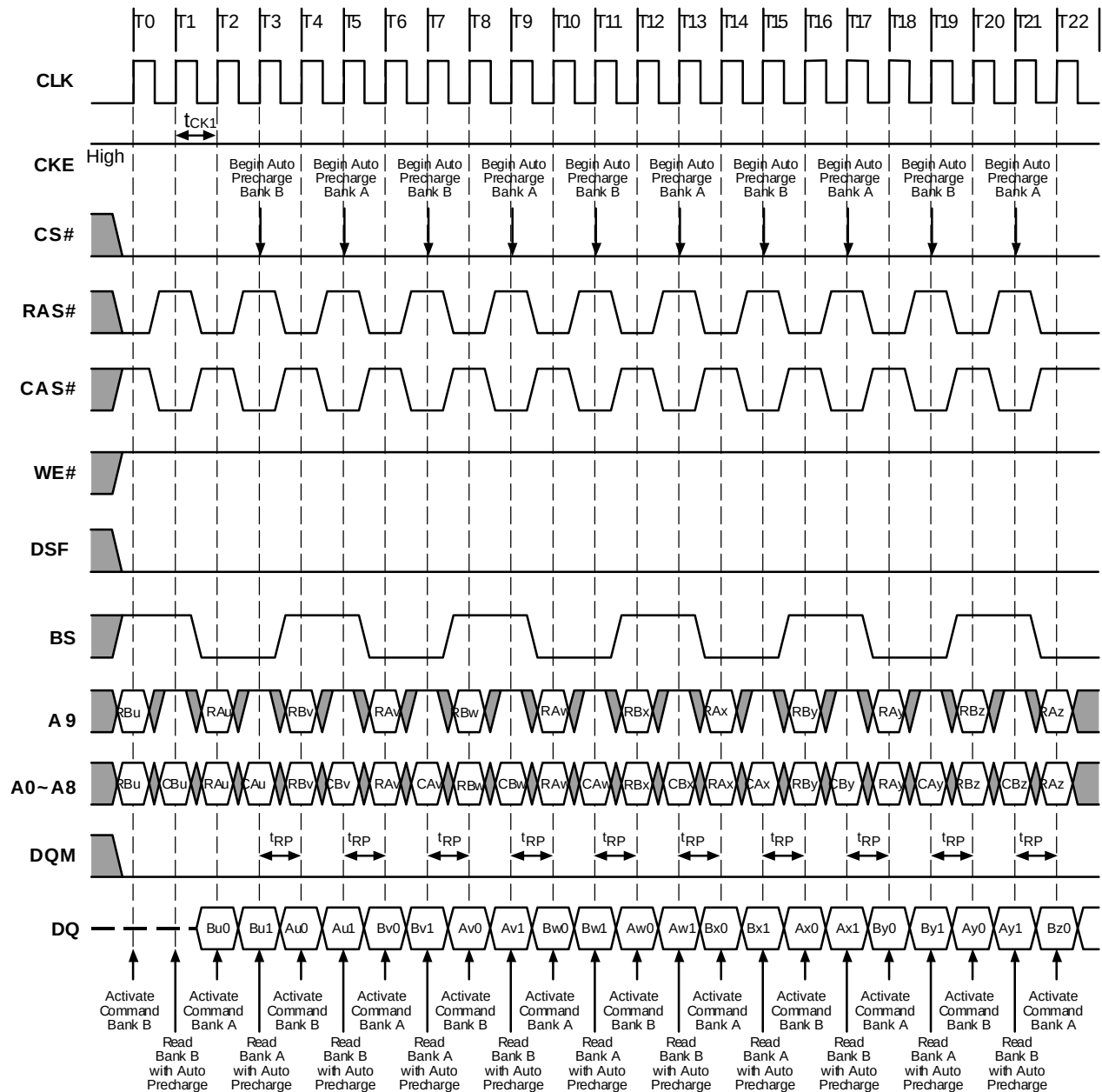
(Burst Length=2, CAS# Latency=1)
