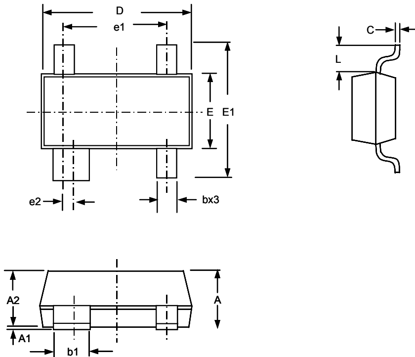
SOT 143 Package
