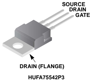
JEDEC TO-220AB
