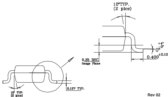
TSOT-23-5 (D5)
