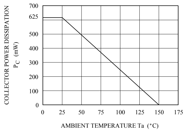
P_C - T_a
