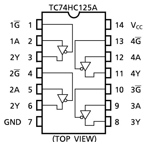
F (SOP14-P-300-1.27) Weight : 0.18g (Typ.)
