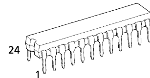
P (DIP24-P-300-2.54) Weight : 1.50g (Typ.)
